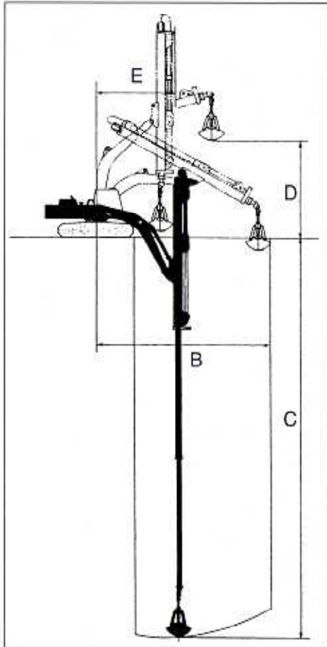
■作業範囲図
