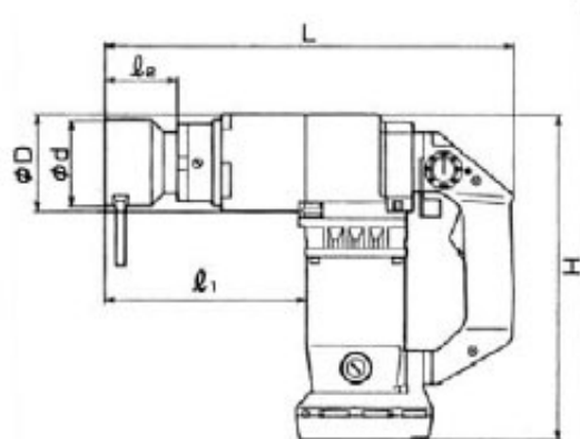
寸法図B
