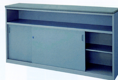
ハイカウンターNED 1200:W1200×D460×H950 1800:W1800×D460×H950
